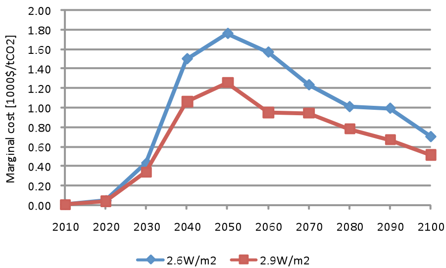
Fig.3-5 CO2 price
